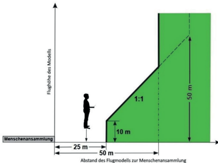
a) Abstandsregeln ohne Sicherheitszaun
